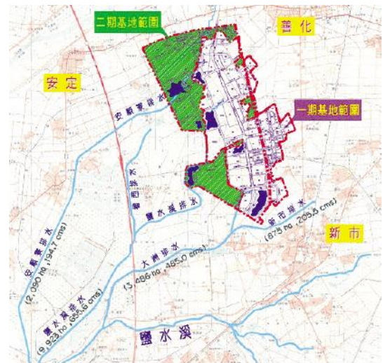
▲ 園區排水系統
