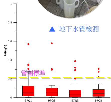
▲ 各季砷離子濃度
