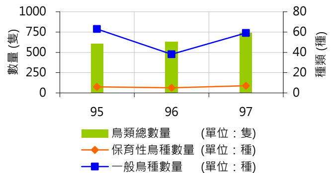
▼ 園區鳥類總數與種類數
