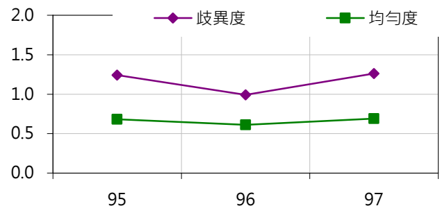
▼ 園區生物多樣性指數(鳥類)
