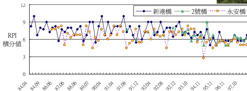
▲ 歷年承受水體 RPI 變化趨勢
