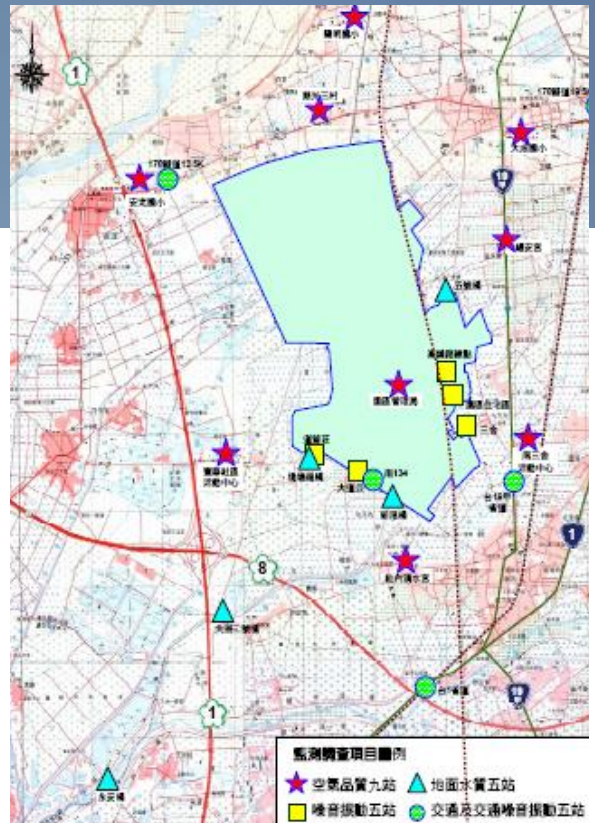
▲ 園區各類環境監測位置
